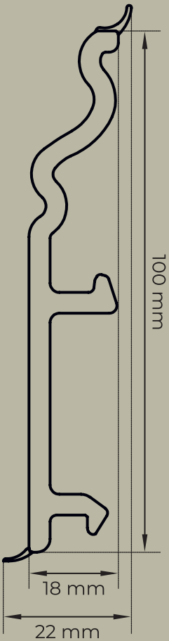
SCALE 1:1
